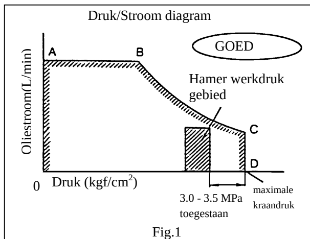
Voorbeeld van Druk/Stroom curve
