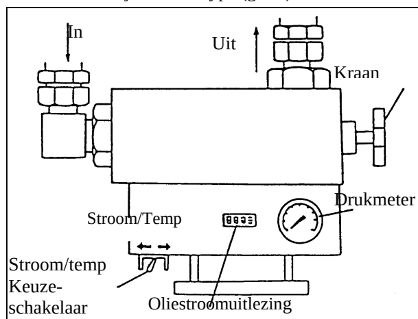
Typische oliestroommeter uitgerust met smoorventiel
